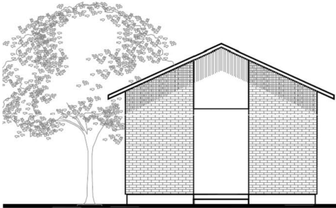
ELEVAÇÃO FRONTAL SEM ESCALA
